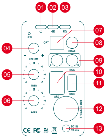
Aktív hangszóró
